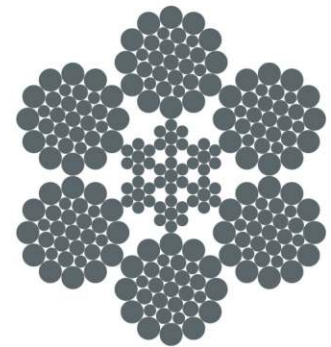
6×31WS-IWRC
