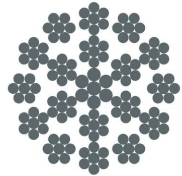
18×7-WSC
