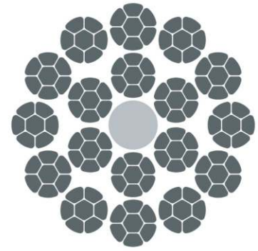
18×K7-FC
