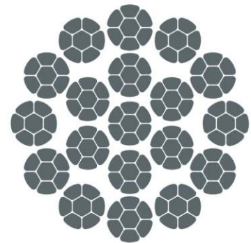
18×K7-WSC
