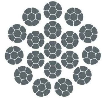
17×K7-WSC
