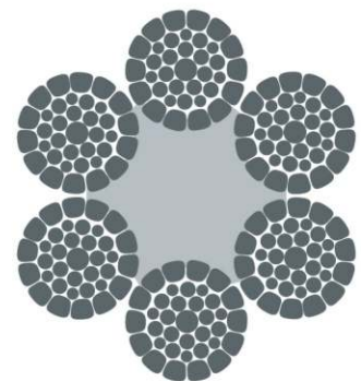
6×K36WS-FC
