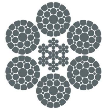
6×K29F-IWRC
