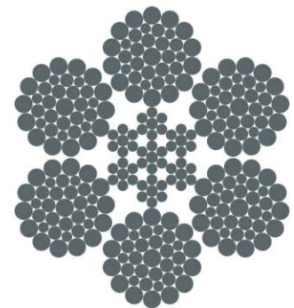
6×36WS-IWRC
