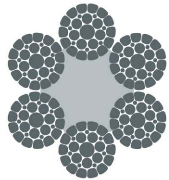
6×K29F-FC
