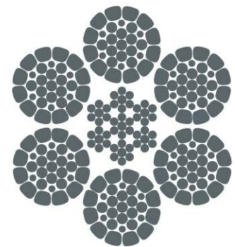
6×K31WS-IWRC
